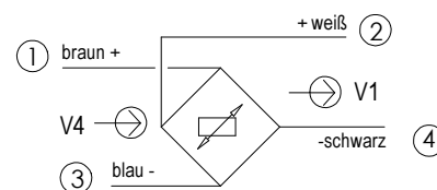
V4: Speisespannung V1: Signalspannung
