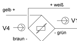
V4: Speisespannung V1: Signalspannung
