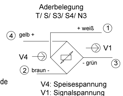
Option S3 Steckverbindung, gewinkelt, M8, angespritzt
