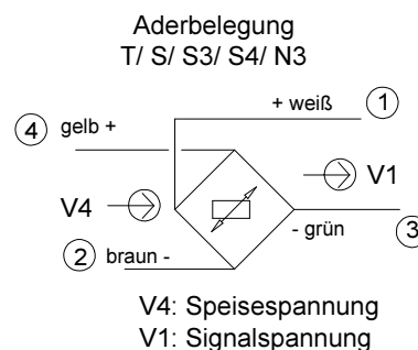
Option S4 Steckverbindung, gewinkelt, C091
