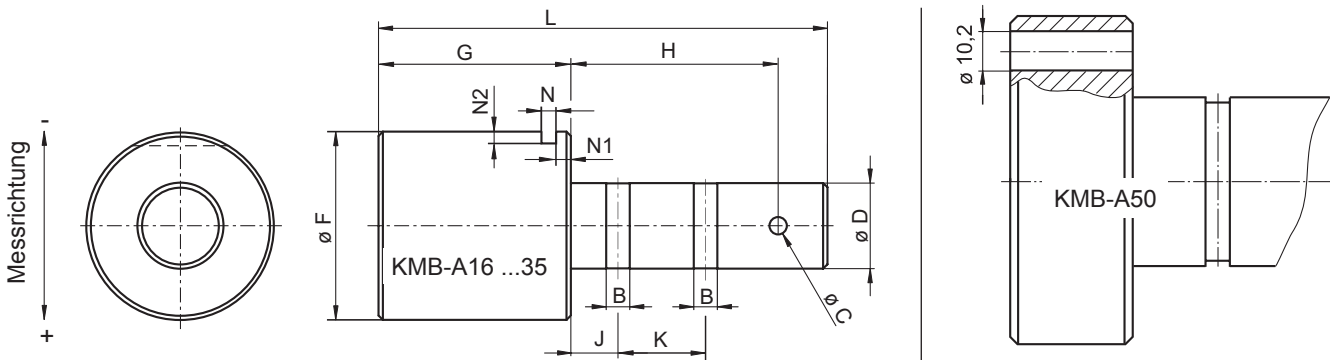
Abmessungen in mm Standard: Kalibrierung im positiven Messbereich, KMB12 ...KMB35 werden auf Zug, KMB50 auf Druck kalibriert
