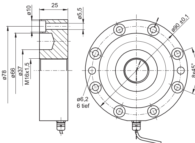
Ausführung D Nennkraft 100; 200 kN
