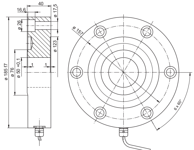
Ausführung E Nennkraft 100, 200 kN
