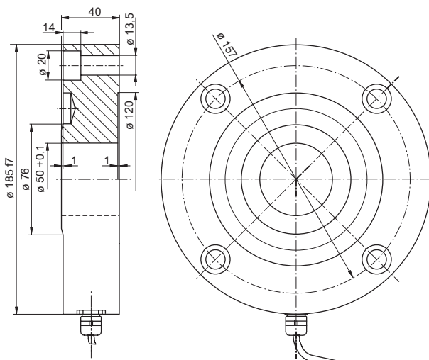
Ausführung D Nennkraft 100; 200 kN
