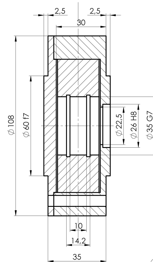
A-A (1:1)
