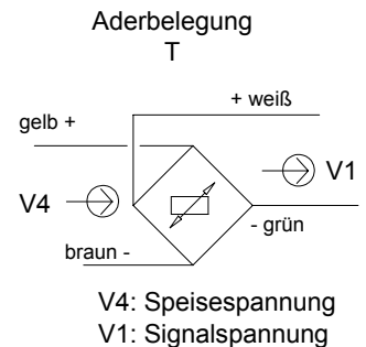
Option T Kabelverschraubung, gerade
