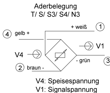
Option N3 Steckverbindung, gerade, M8, angespritzt
